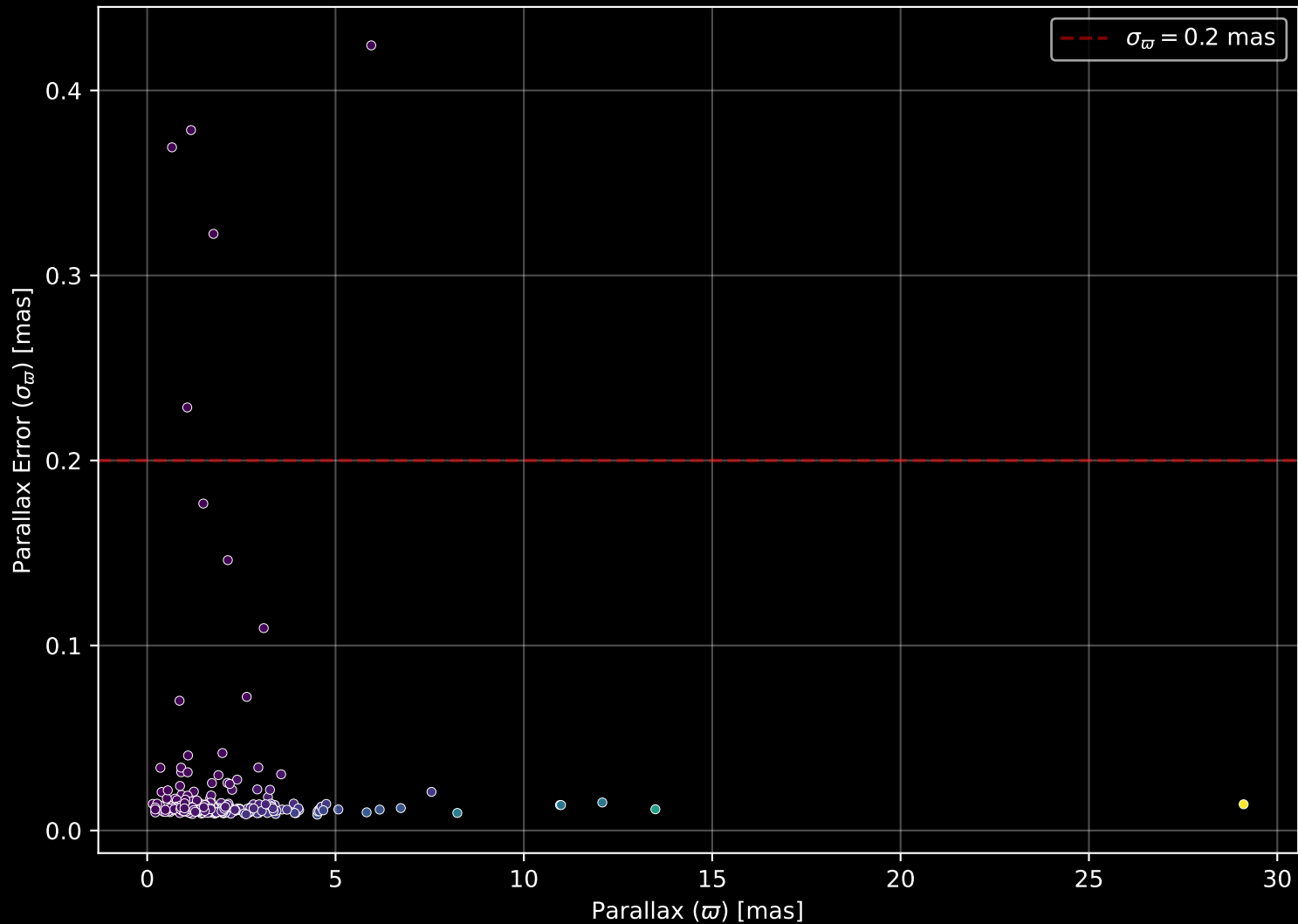
GALAH DR4 Field: [7041] Parallax Quality (n= 291)
