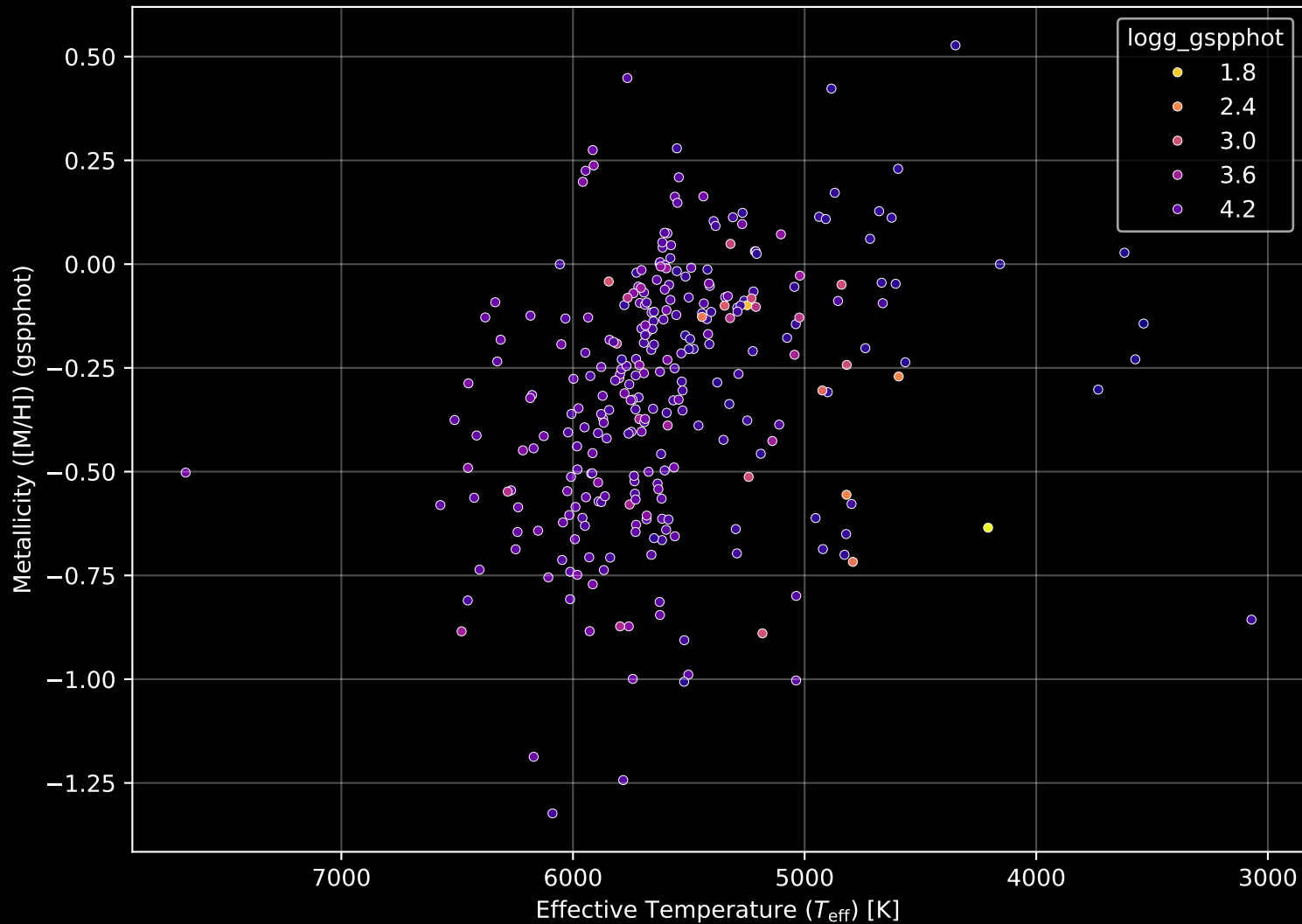
GALAH DR4 Field: [7041] Stellar Population Parameters (n= 291)
