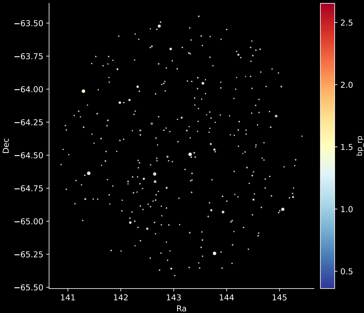
GALAH DR4 Field: [7041] Stars: 291
